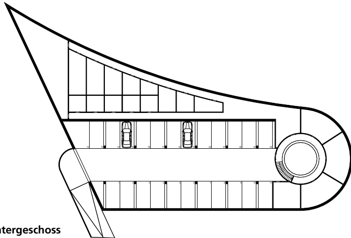
Erdgeschoss
