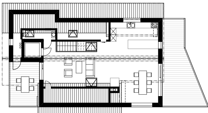
Dachgeschoss
